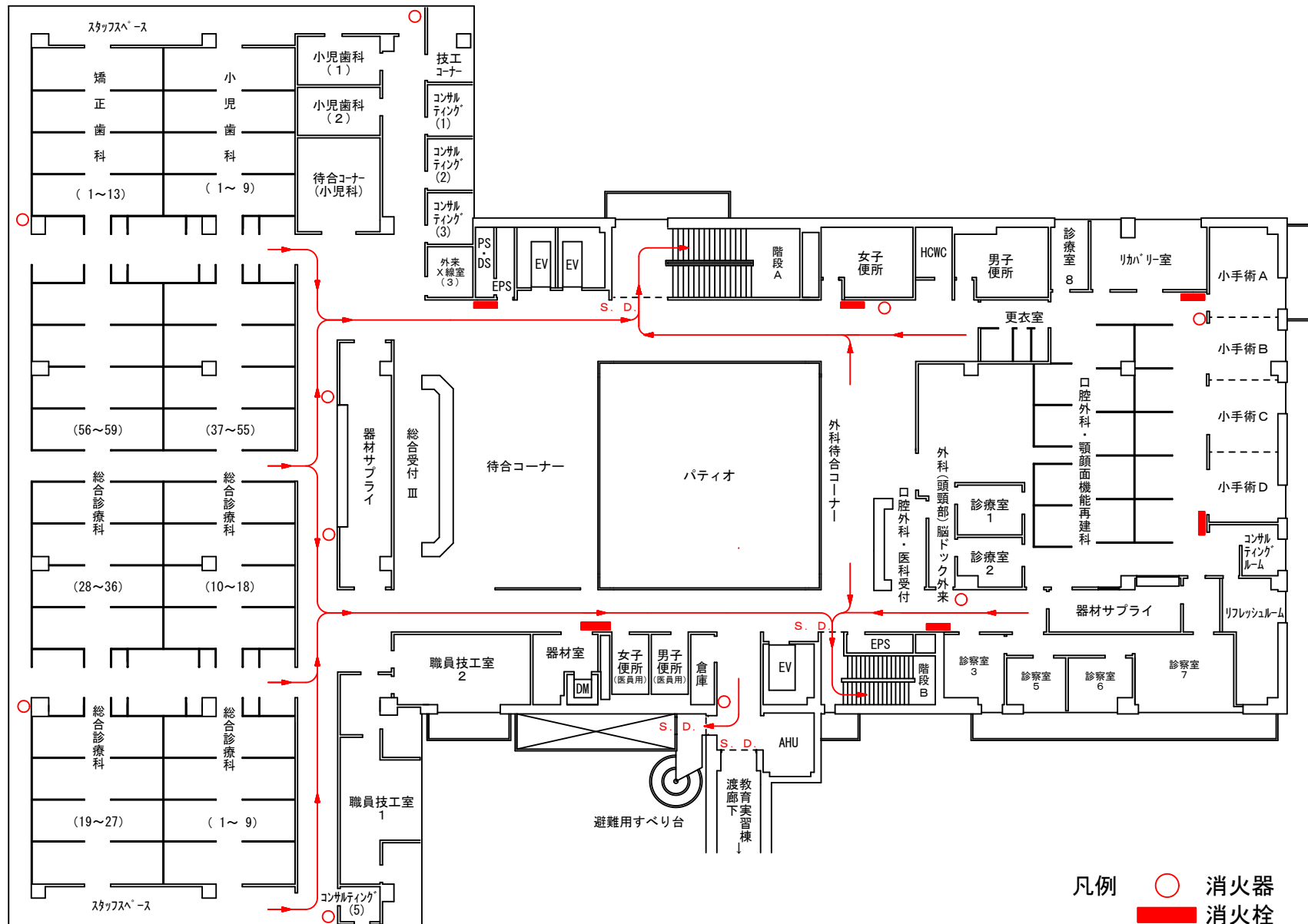
付属病院棟 3階平面図
