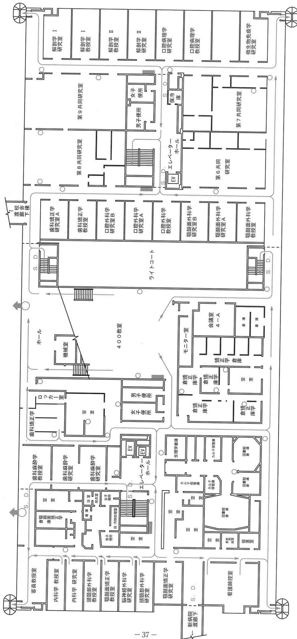
4 階 平 面 図
